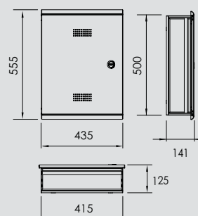
Caixa vazia embutir M2AT
