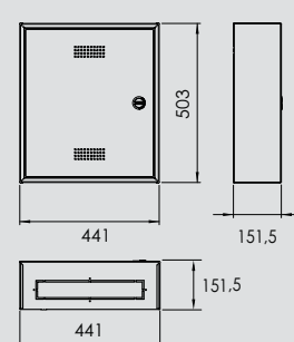
Caixa vazia saliente I3SM2AT
