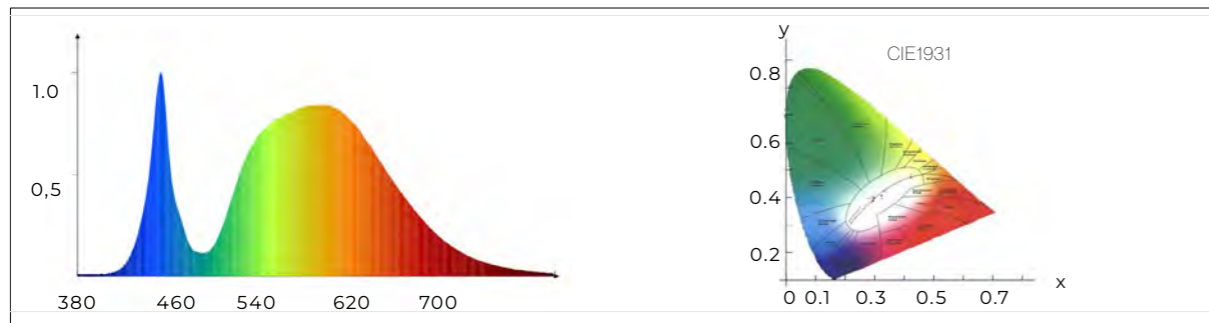
ESPECTRO FOTOMÉTRICO
