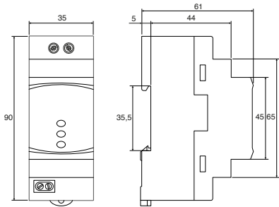
CEM-M
