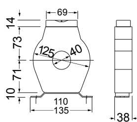
TRM140
