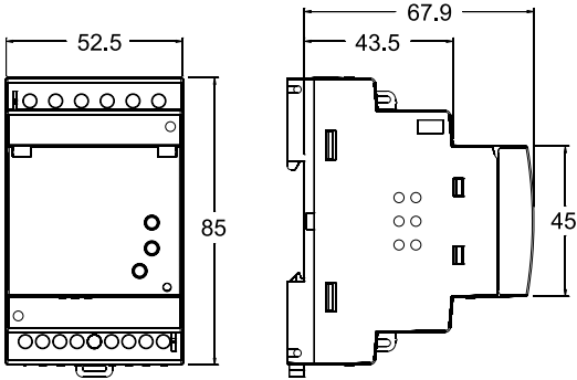
CVM NET
