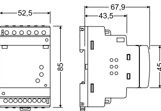
RECmax CVM
