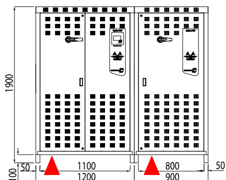
OPTIM 14L
