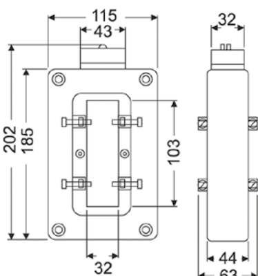
TA 500
