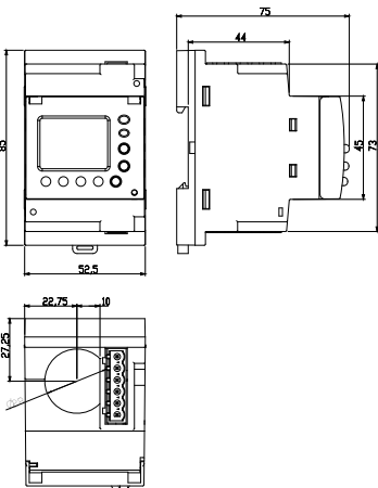
WRU-10
