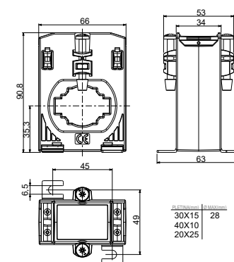
TD 6
