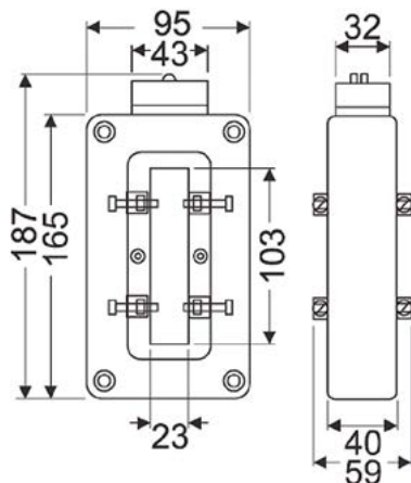
TA 210
