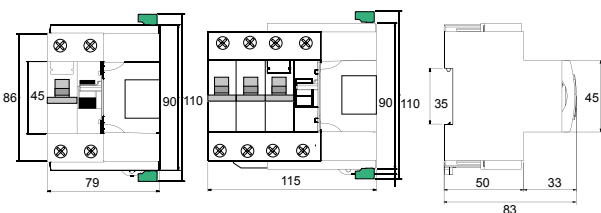
RECmax
