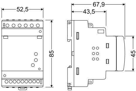
WRU-10
