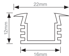
Perfil de Encastrar Alto High Recessed Aluminium Profile Profilé Encastré haut en Aluminium
