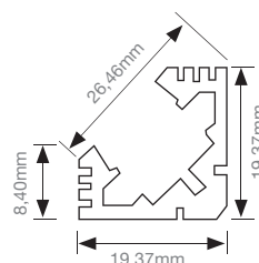
Perfil de canto Corner Profile Profilé d'angle 90°
