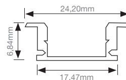
Perfil de Encastrar Baixo Low Recessed Aluminium Profile Profilé Encastré bas en Aluminium
